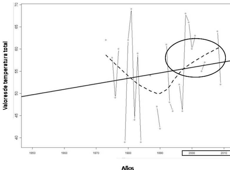
Figura 2: Comportamiento estadístico de la media móvil para los valores de temperatura en la estación San Vicente.
