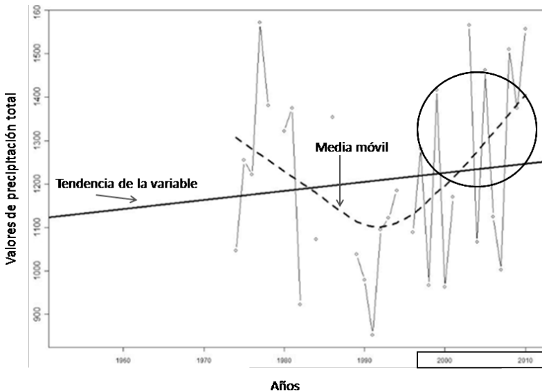
Figura 1: Comportamiento estadístico de la media móvil para los valores de precipitación total en la estación Lebrija, aeropuerto Palo Negro.
