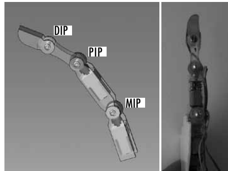
Figura 2. Dedo antropomórfico (diseño CAD y dedo real)
