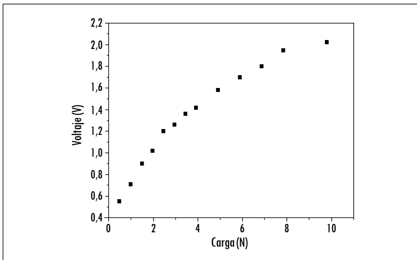
Figura 6. Curva de calibración del FSR
