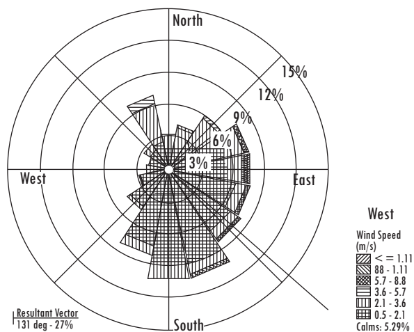
Figura 6. Rosa de los vientos del área de interés, 2007
