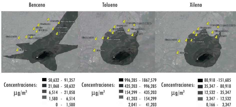
Figura 5. Concentraciones en los receptores de benceno, tolueno y xileno para 2007, al aumentar la emisión en un orden de magnitud
