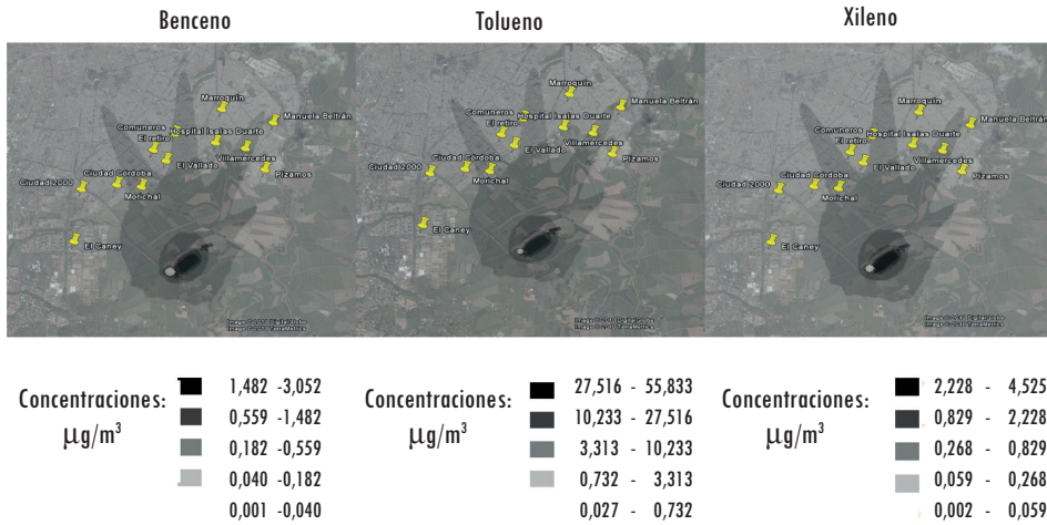
Figura 4. Concentraciones en los receptores de benceno, tolueno y xileno para 2007, al disminuir la emisión en un orden de magnitud
