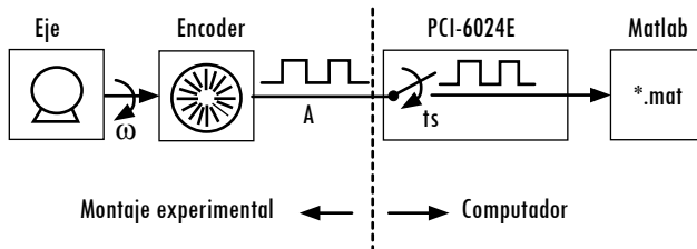
Figura 10. Montaje experimental y procesamiento de las señales
