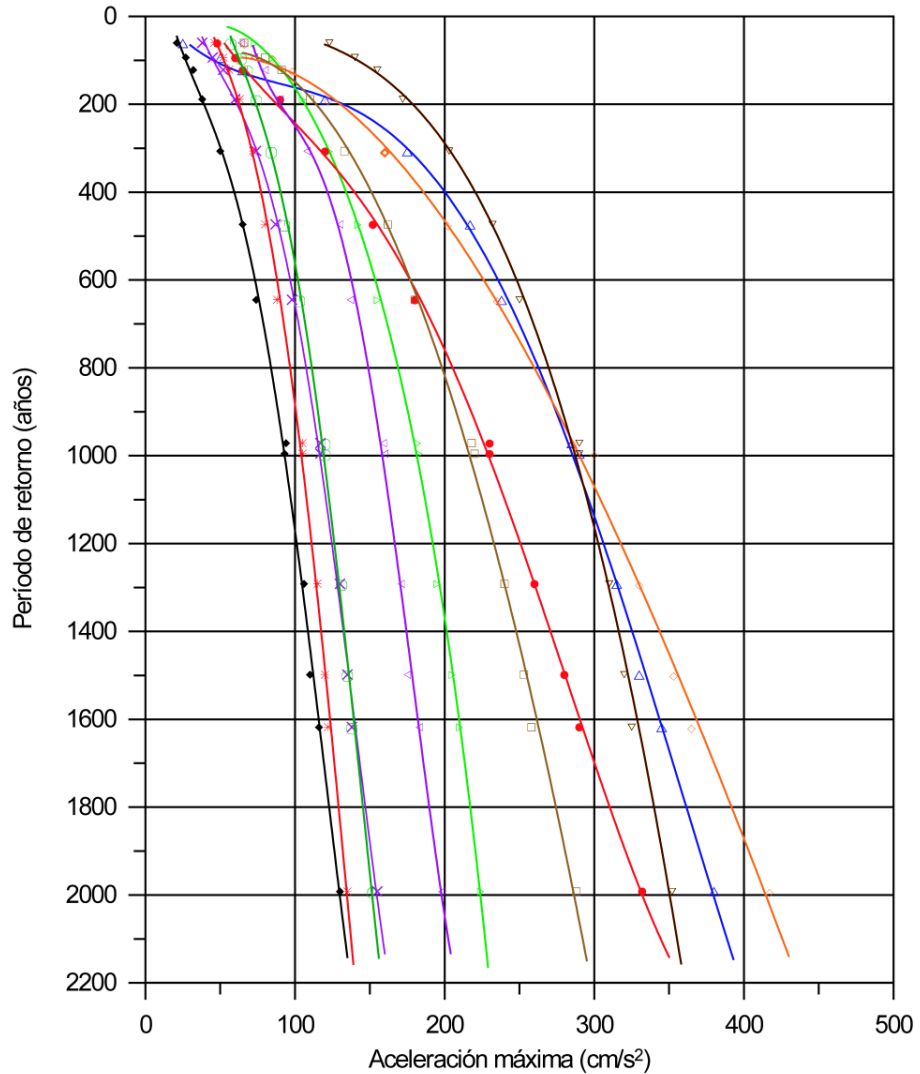
Figura 6. Aceleración máxima probable a_{m\acute{a}x} para diversos valores del periodo de retorno promedio T_R
