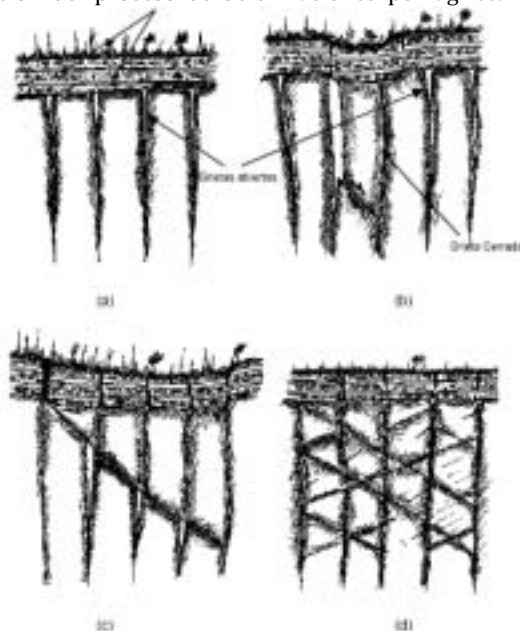
Figura 1. Ilustración del proceso de deformaciones por agrietamiento.
