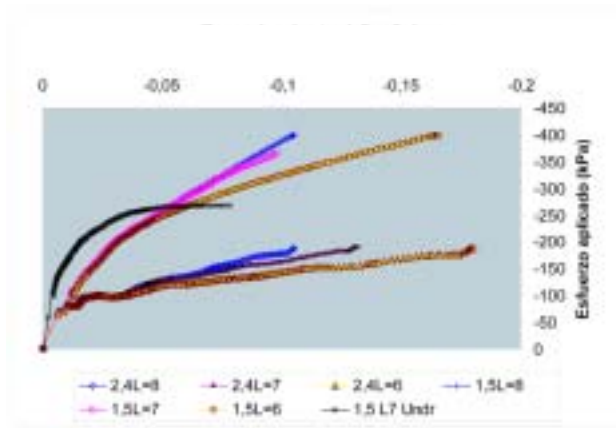
Figura 15. Efecto del refuerzo con columnas de suelo-cemento-cal en función de su longitud (L) y el espaciamiento sobre las cargas admisibles y los asentamientos para condición drenada (cargas permanentes a largo plazo, y no drenada -Undr- para las columnas de 1,5m de separación y 7 m de longitud).
