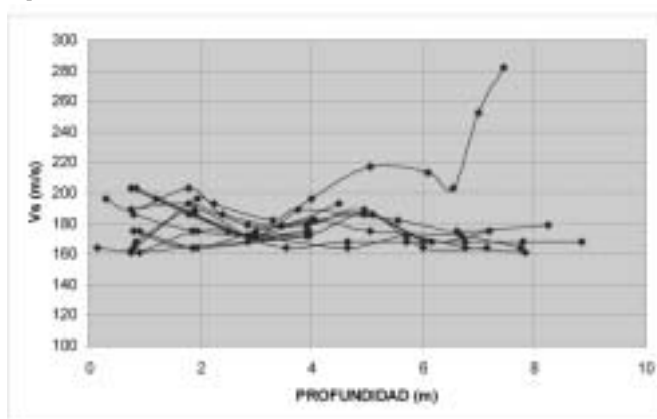
Figura 8. Variación de la velocidad de onda de corte ( V_s ) con la profundidad estimada a partir de los valores de SPT.
