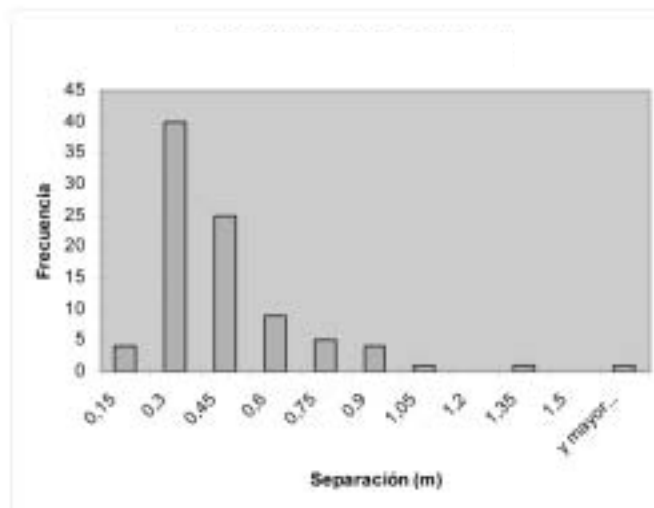
Figura 3. Histograma de separación de grietas
