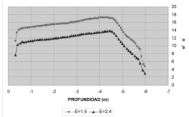
Figura 16. Distribución de esfuerzos de compresión a lo largo de las columnas de suelo estabilizado para separación de E=1,5 m y E=2,4 m entre columnas, condición drenada (cargas permanentes a largo plazo).
