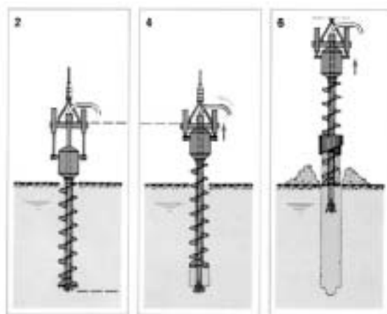
Figura 17 Esquema constructivo para las columnas de suelo estabilizado con cal y cemento.
