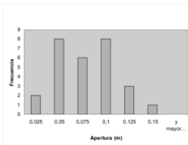
Figura 2. Histograma de apertura de grietas
