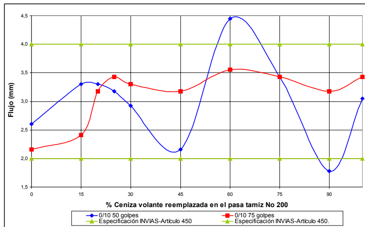
Figura 5. Variación del flujo con respecto al reemplazo de ceniza en el tamiz pasa número 200
