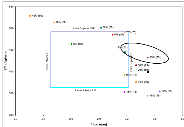
Figura 6. Variación de la relación estabilidad-flujo
