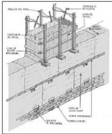
Figuras 28 y 29: Esquema de la construcción de una edificación en tapia pisada
