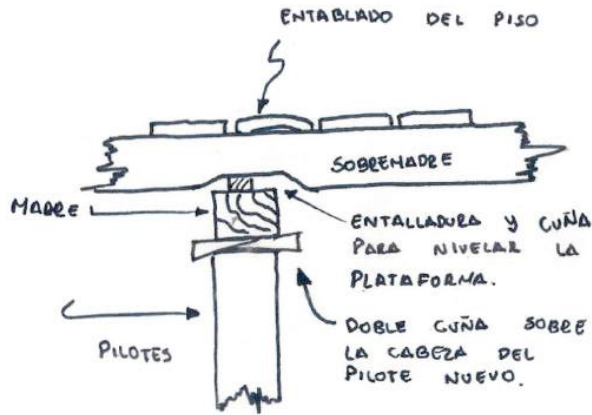
Figura 10: Detalle del remplazo de los pilotes deteriorados y como se adhieren a la estructura existente Fuente: Modificado de Mallol y De Recasens, 1963
