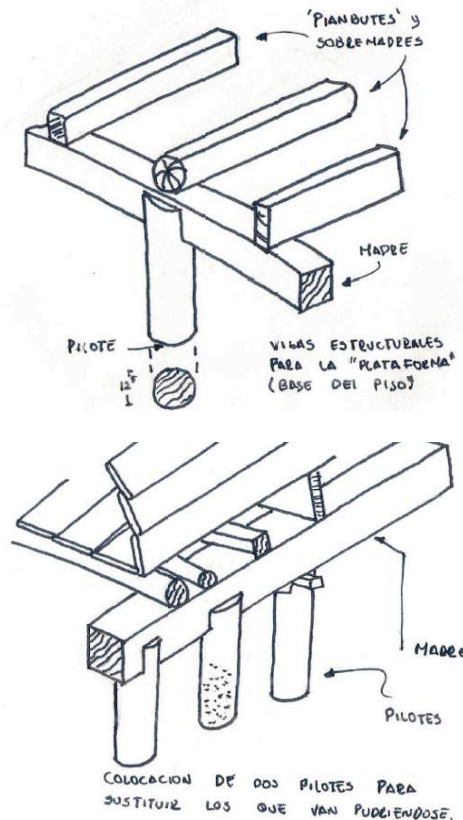
Figura 9: Diagrama de colocación de los pilotes (arriba) y estructura de piso (abajo) Fuente: Modificado de Mallol y De Recasens, 1963
