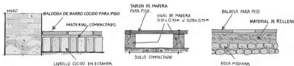
Figura 27: Distintas configuraciones para pisos de construcciones en tapia pisada
