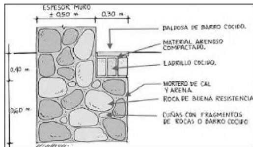
Figuras 25 y 26: Viga de cimentación y sobrecimiento
