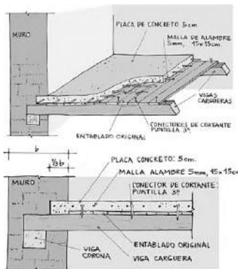
Figuras 30 y 31: Detalles para garantizar la acción de diafragma mediante la losa
